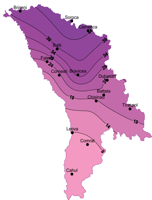
Fig.3. Riscul vătămării soiurilor de viță de vie relativ rezistente la ger (probabilitatea %, T < -22\text{ }^{\circ}\text{C} ) pe teritoriul Republicii Moldova
