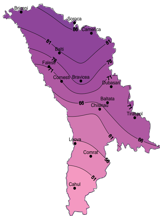
Fig.2. Riscul vătămării soiurilor de viță de vie sensibile la ger (probabilitatea %, T < -17\text{ }^{\circ}\text{C} ) pe teritoriul Republicii Moldova
