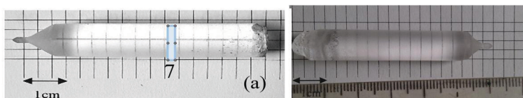
Figura 2. Cristale de (a) \text{BaF}_2:0.1 \text{ mol\% ErF}_3 , respectiv (b) \text{CaF}_2:0.1 \text{ mol\% ErF}_3 obținute în cadrul Laboratorului de Creștere a Cristalelor de la Facultatea de Fizică a UVT.
