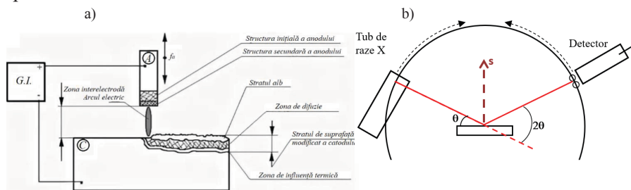
Fig.1. Reprezentarea schematică a procesului ASE a) și reprezentarea schematică a modului de măsurare \theta - 2\theta în geometria de focalizare Bragg-Brentano b)
