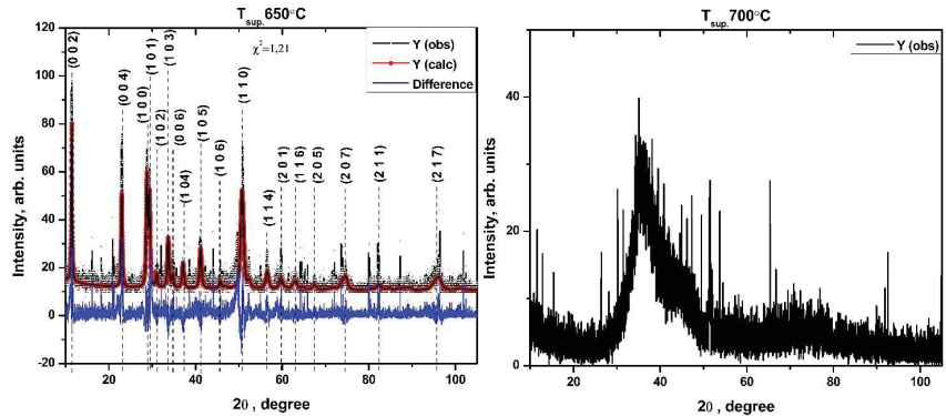
Fig.4. Difractograma și rezultatul Rietveld refinement-ului pentru probele cu temperatura suportului de 650°C și tabloul de difracție pentru proba cu temperatura suportului de 700°C
