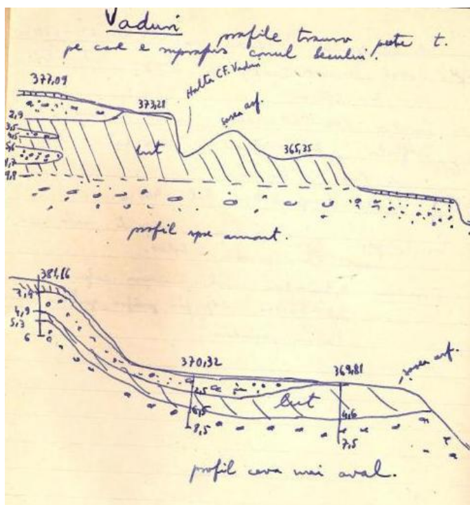
Profile transversale pe Bistrița, la Vaduri (nedatate).
