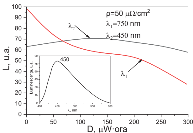
Fig. 6. Dependența intensităților benzilor cu maxime de intensitate centrate la lungimile de undă \lambda_1=450 \text{ nm} și \lambda_2=750 \text{ nm} din spectrul de FL a probei și, respectiv, de reflexie a radiației incidente pe eșantionul respectiv. (Inset) Spectrul FL a frunzei de smochin.
