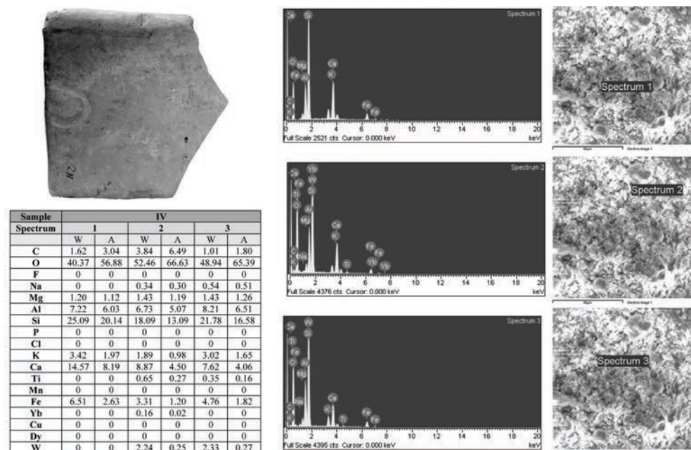
Fig. 6. Eșantionul IV, rezultatele analizei unei țigle de la Sobari.
