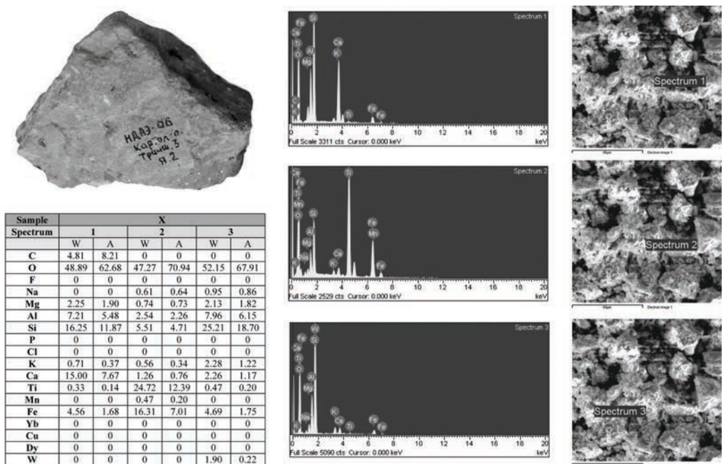
Fig. 12. Eșantionul X, rezultatele analizei unei cărămizi ștampilate de la Cartal-Aliobrix.
