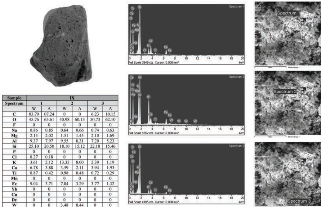
Fig. 11. Eșantionul IX, rezultatele analizei unei țigle de la Cartal-Aliobrix.
