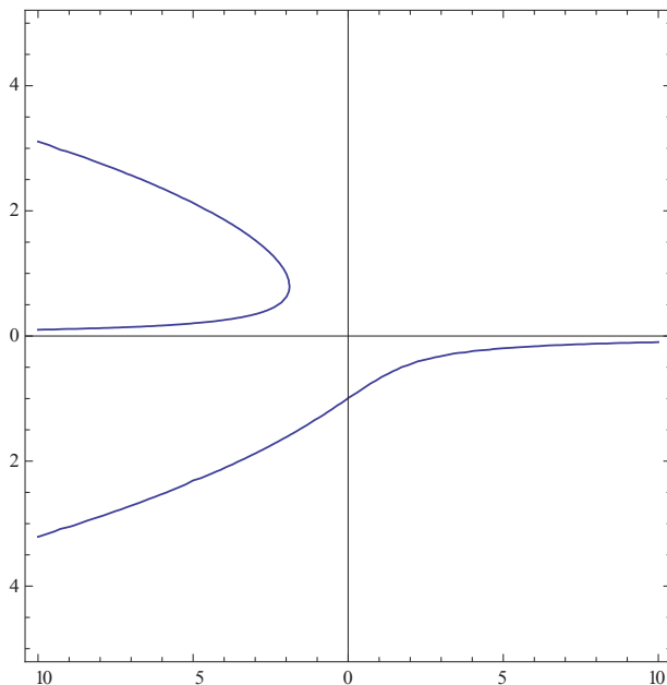
Рис. 3.1. Графическое представление решений кубического уравнения.
