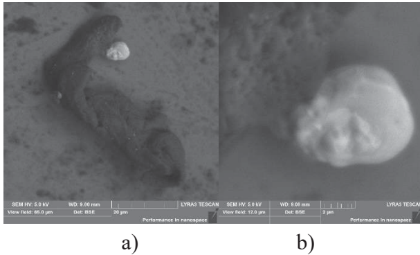
Fig. 2. Particulă de oxid de plumb fotografiată la vid scăzut și la diferite mărituri în modul de înregistrare a electronilor reflectați.
